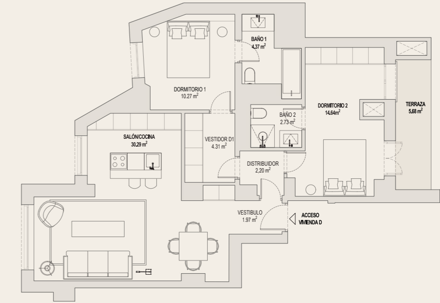
D Superficie construida 124,79 m 2
